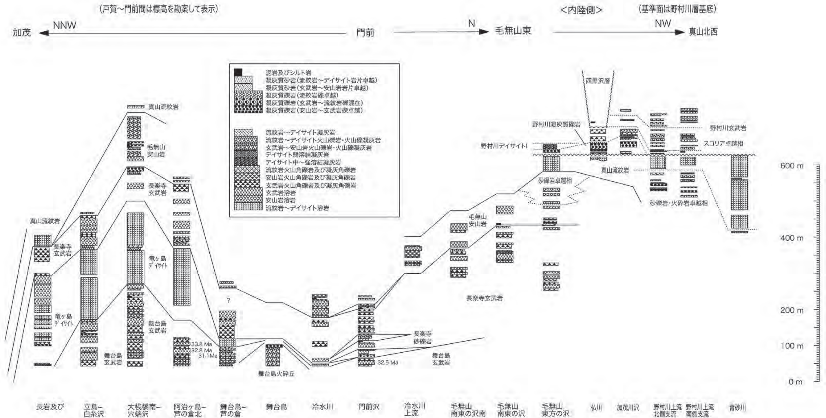
第 4B 図 戸賀湾南側の地域における門前層地質柱状図.
