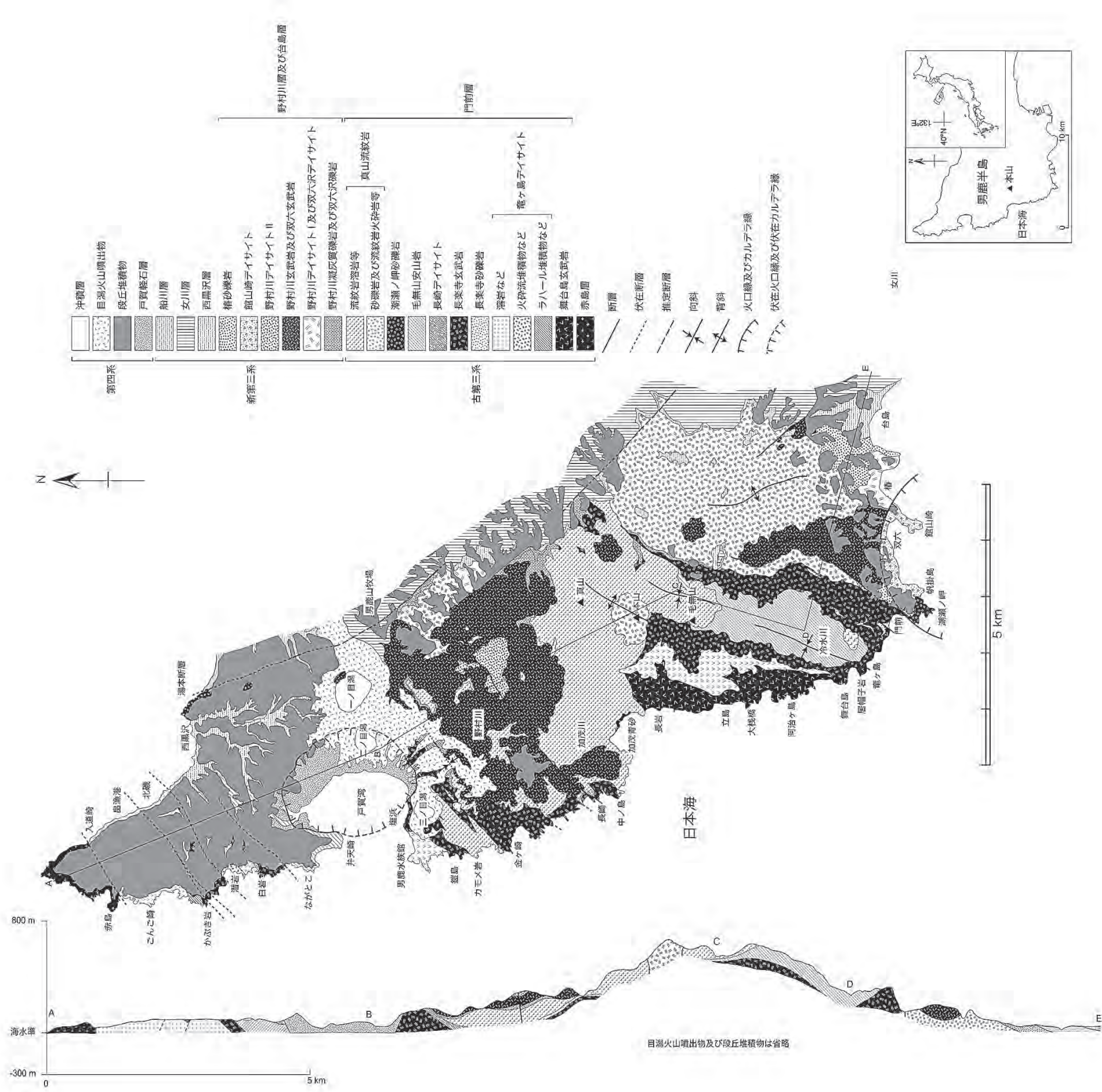
第1図 男鹿半島西部の地質図。台島層と潮瀬ノ岬砂礫岩の地質図は Sato (2006MS) による。
