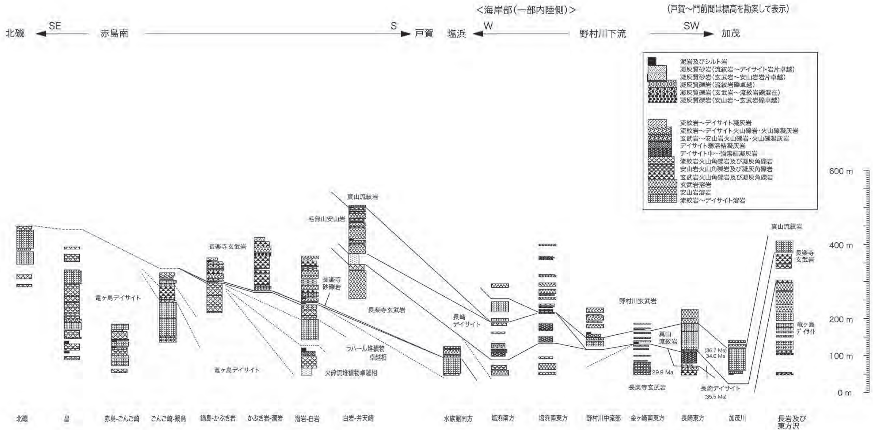
第 4A 図 戸賀湾北側の地域における門前層地質柱状図.
