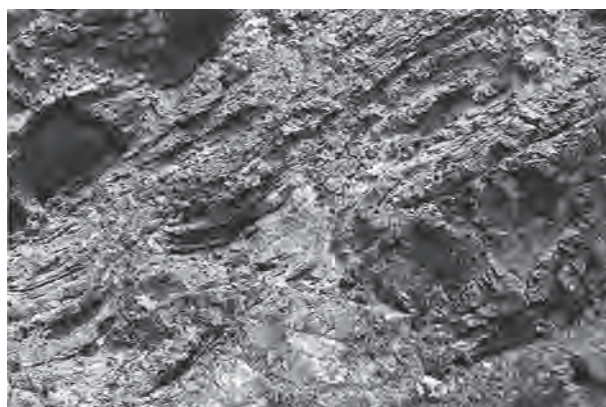
第12図 長崎デイサイトを構成するデイサイト火砕流堆積物（きららかホテル北方、長崎）。溶結し局所的に褶曲している。ハンマーの長さは30 cm。
