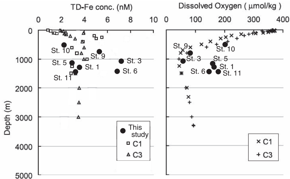
図3 Nishioka et al.(2007) の全可溶鉄量と DO の鉛直分布と本研究の結果.
