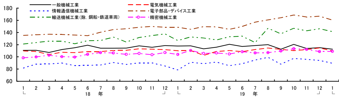
機械工業関係の業種別生産指数
