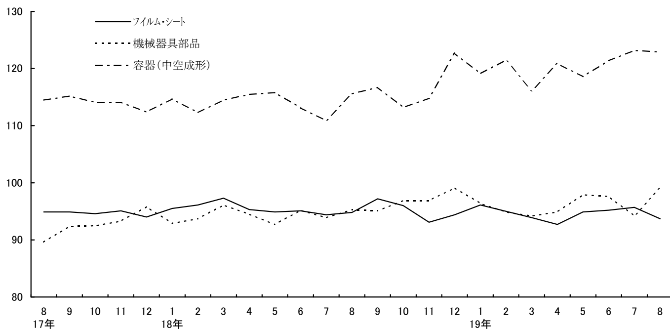
(2) 主要品目別生産指数の推移 (平成12年=100, 季節調整済)
