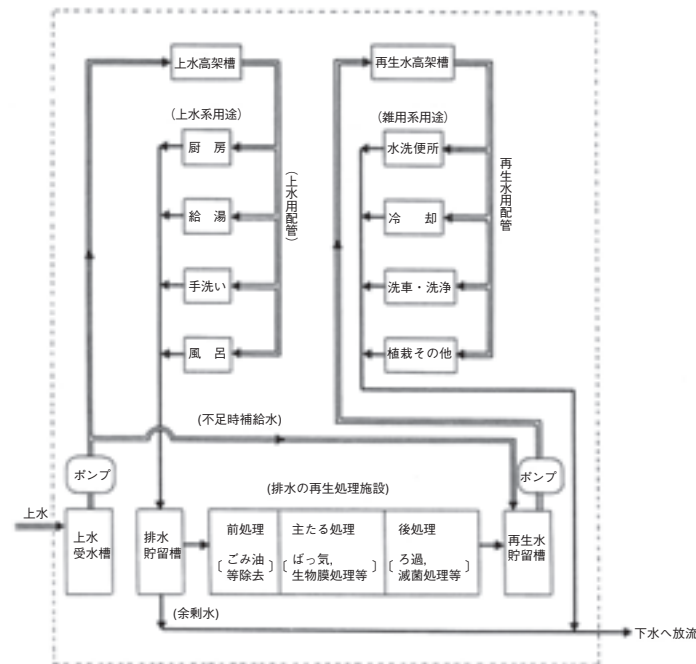
図8－1－2 再生水利用のシステム例
