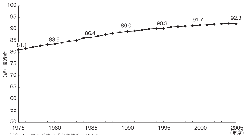
図8－1－1 上水道の有効率の推移
