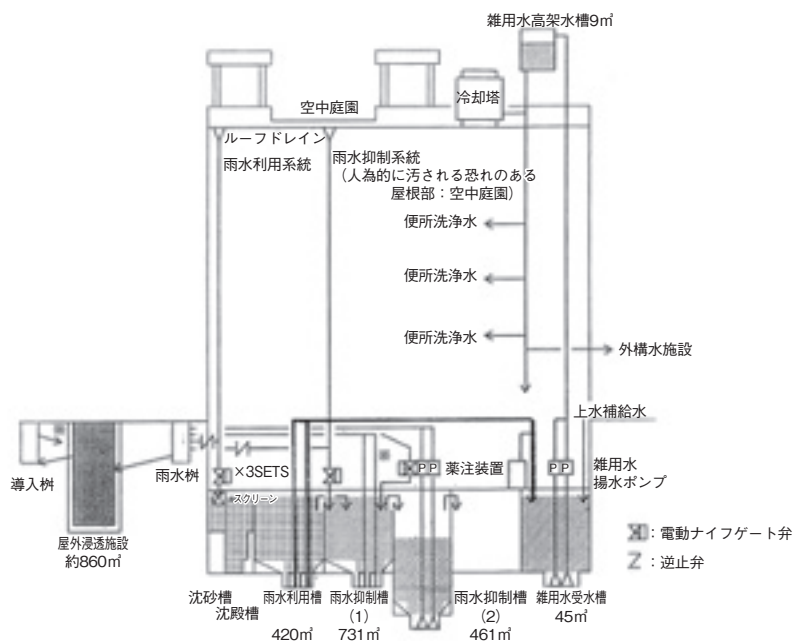
図8-1-5 雨水利用の事例（綾瀬市庁舎（神奈川県）配水系統図）
