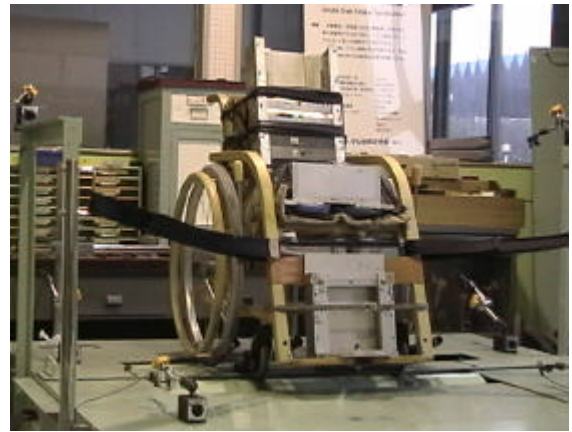
Fig.2 竹製車椅子の走行耐久性試験
