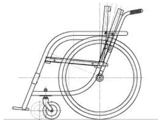
Fig.7 竹製車椅子の主要構造
