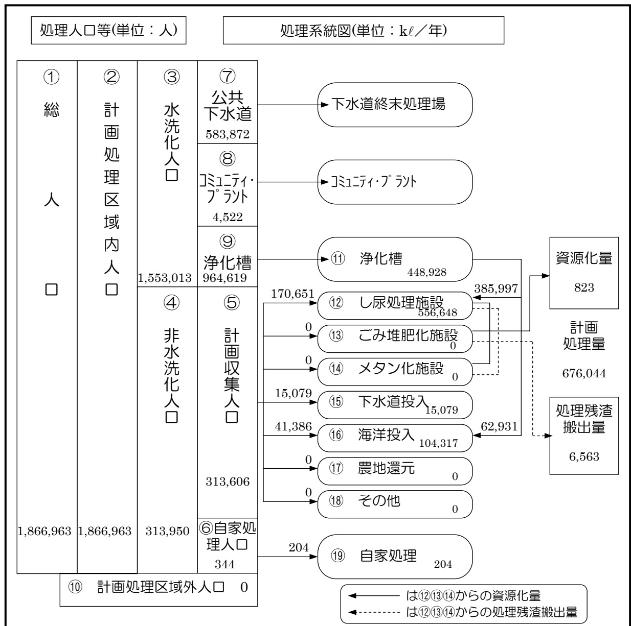
資料7-11 し尿処理のフロー図（平成17年度）
