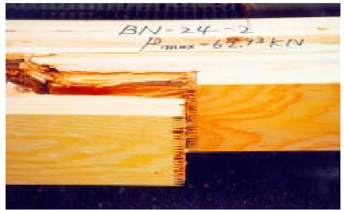
図6 フィンガージョイント部の破壊
