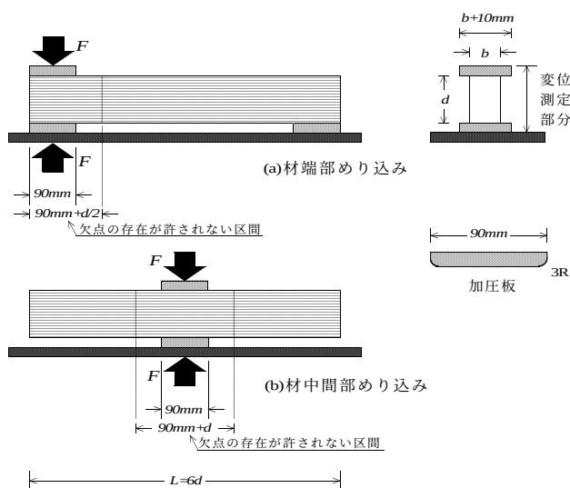
図3 めり込み試験方法
