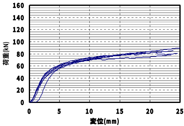
図7 荷重－変位曲線（B-21端部）
