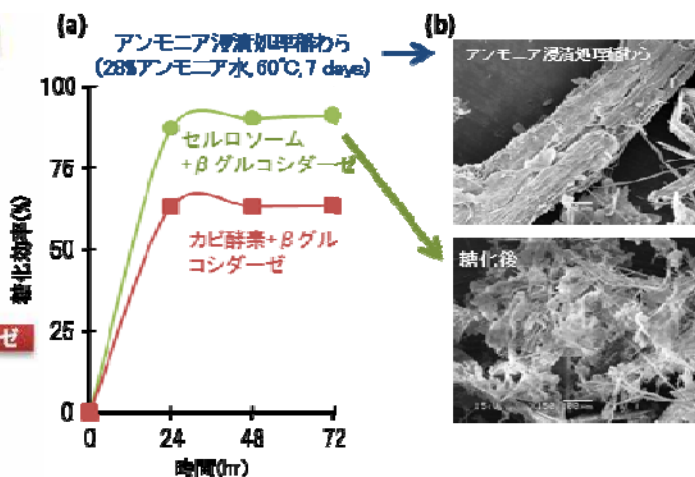
図3 セルロソームと T. Brockii 由来βグルコシダーゼ酵素ミックスを用いた稲わら糖化 (a)；アンモニア浸漬処理稲わらの糖化。(b)；稲わら糖化後のSEM画像。酵素はそれぞれ 1 g 基質あたり 2 mg 使用した。
