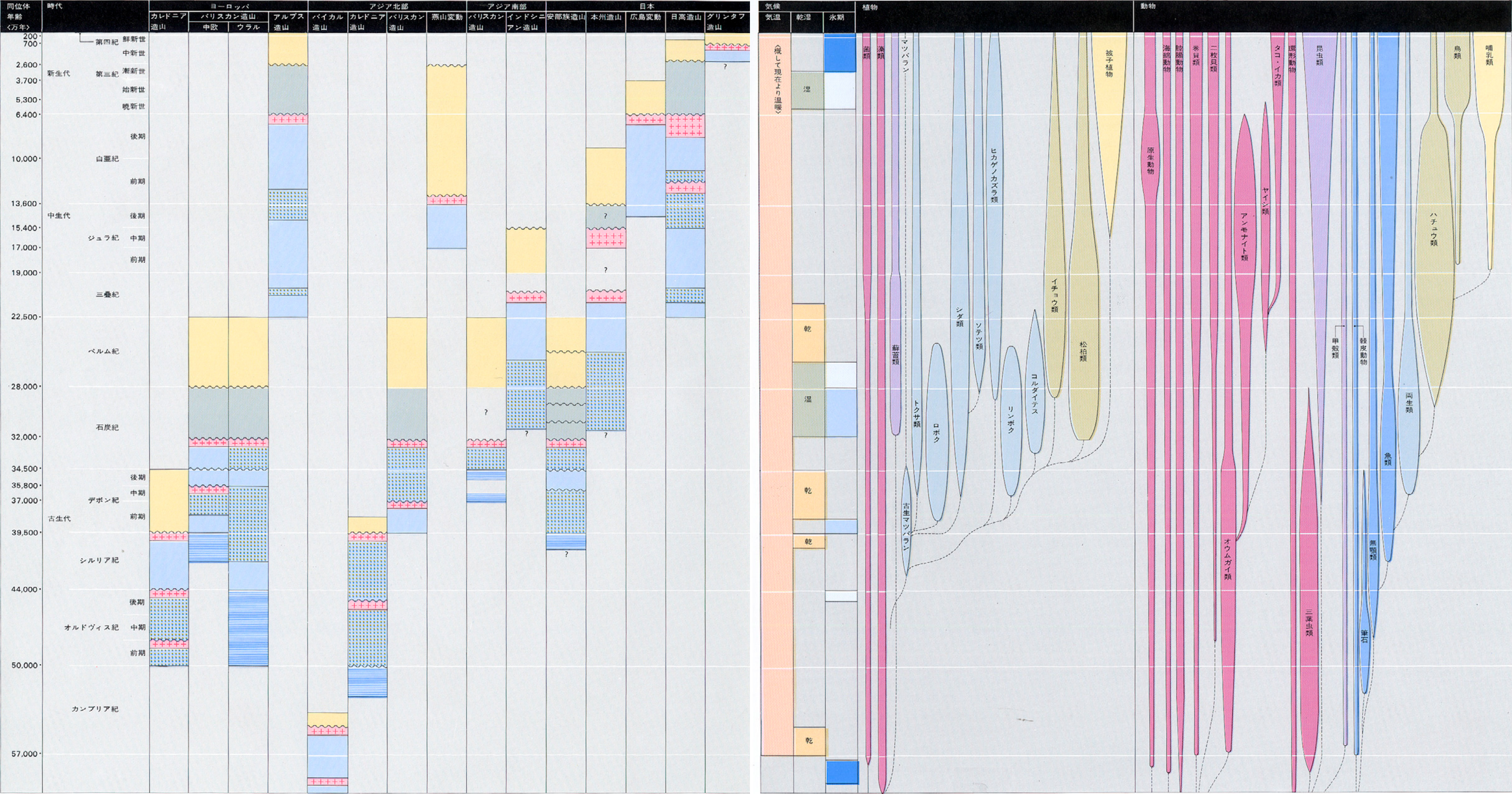
図4・2 - 造山帯と造山運動の過程
