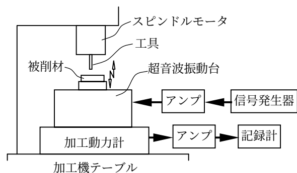
Fig.7 穴加工実験
