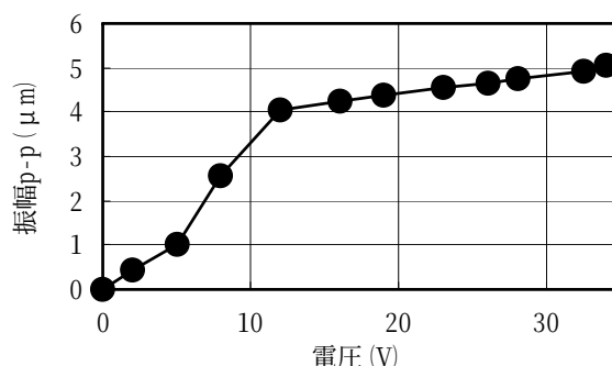
Fig.3 電圧と振幅の関係
