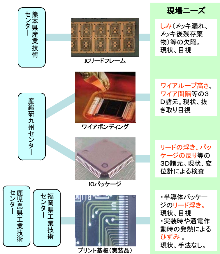
図1 役割連携のイメージ(高精度・高スループット2D-3Dインスペクション技術の開発)
