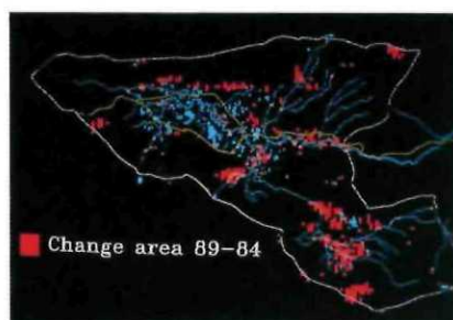
写真－3 雨竜沼湿原を対象に、1984年と1989年の画像を重ね合わせて5年間の変化を抽出した写真 赤が湿原からササ地に变化したと判断された箇所
