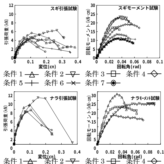
Fig.4 ほぞ試験結果
