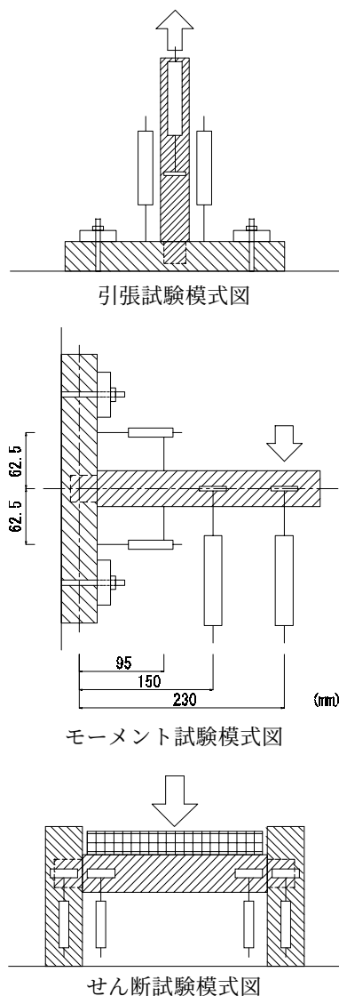
Fig.2 ほぞ試験体の試験方法
