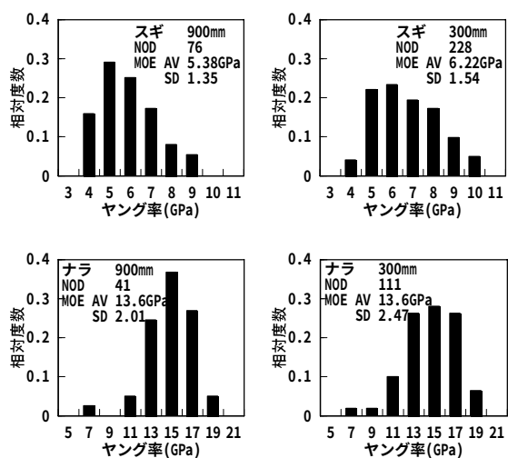
Fig.3 縦振動法で測定した 900mm および 300mm のスギ、ナラのヤング率の分布
