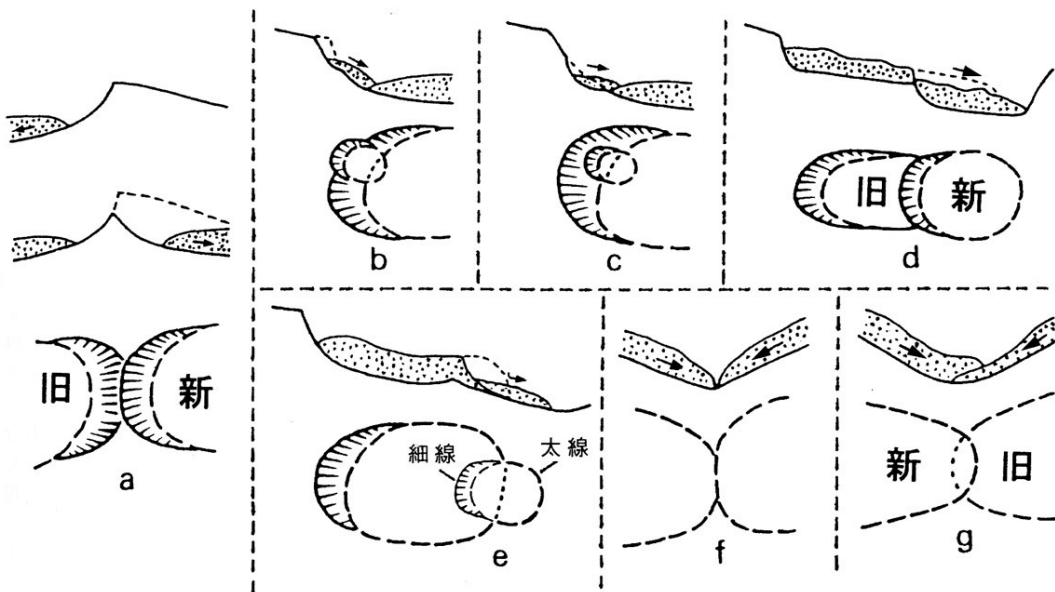
図2 複数の地すべり地形の相互関係とその表現方法 (旧: より古い地すべり地形, 新: より新しい地すべり地形) Fig. 2 Mutual relationship of overlapping landslides and expression method (Old: Older landslide, New: Newer landslide).
