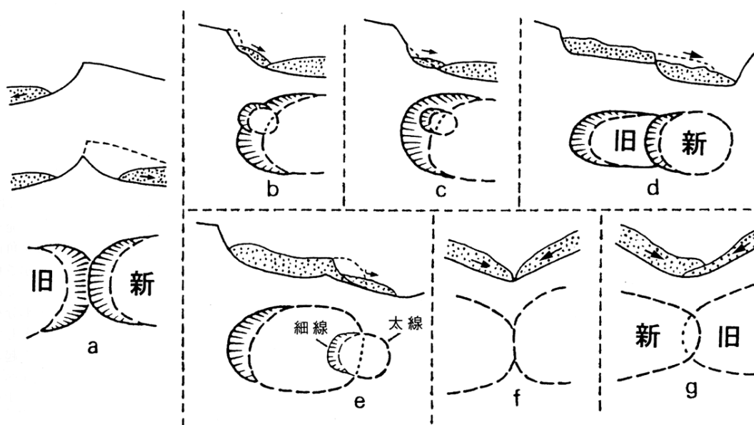
図2 複数の地すべり地形の相互関係とその表現方法 (旧: より古い地すべり地形, 新: より新しい地すべり地形)
