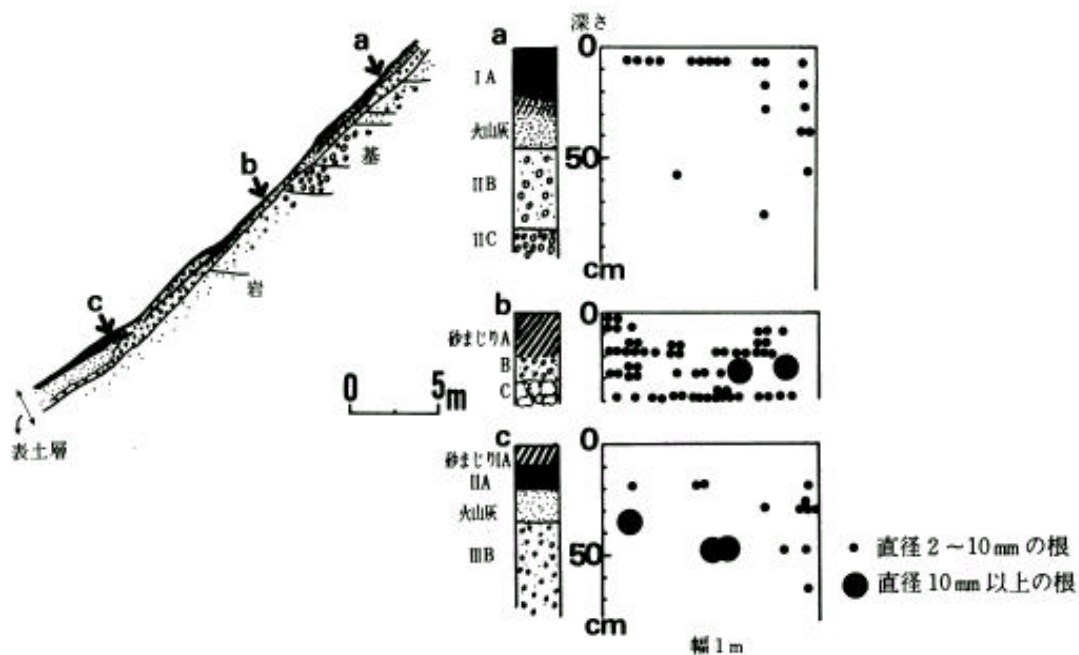
図 - 4 表土層の根系の分布
