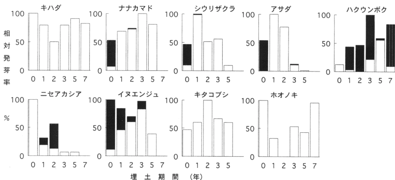
図 - 4 タイプ3：発芽率の低下が明瞭ではない樹種の相対発芽率の推移
