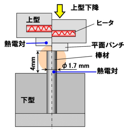
図1 金型構造の概略
