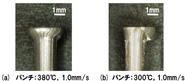
図4 温度条件による成形品形状の差
