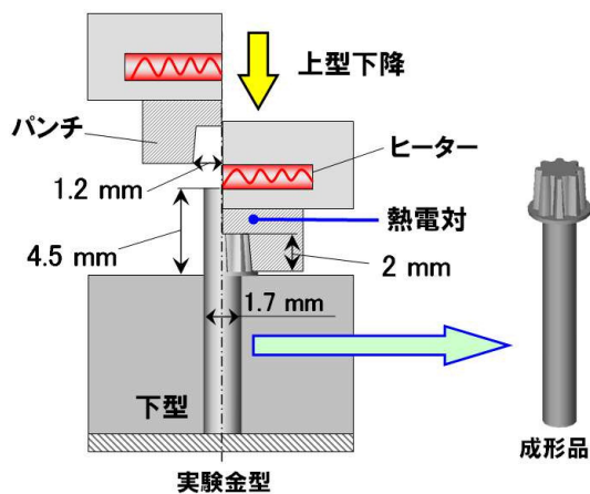
図7 金型概略図
