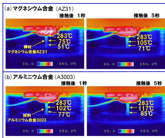
図2 温度分布測定結果
