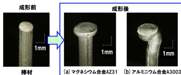
図3 成形前後の外観
