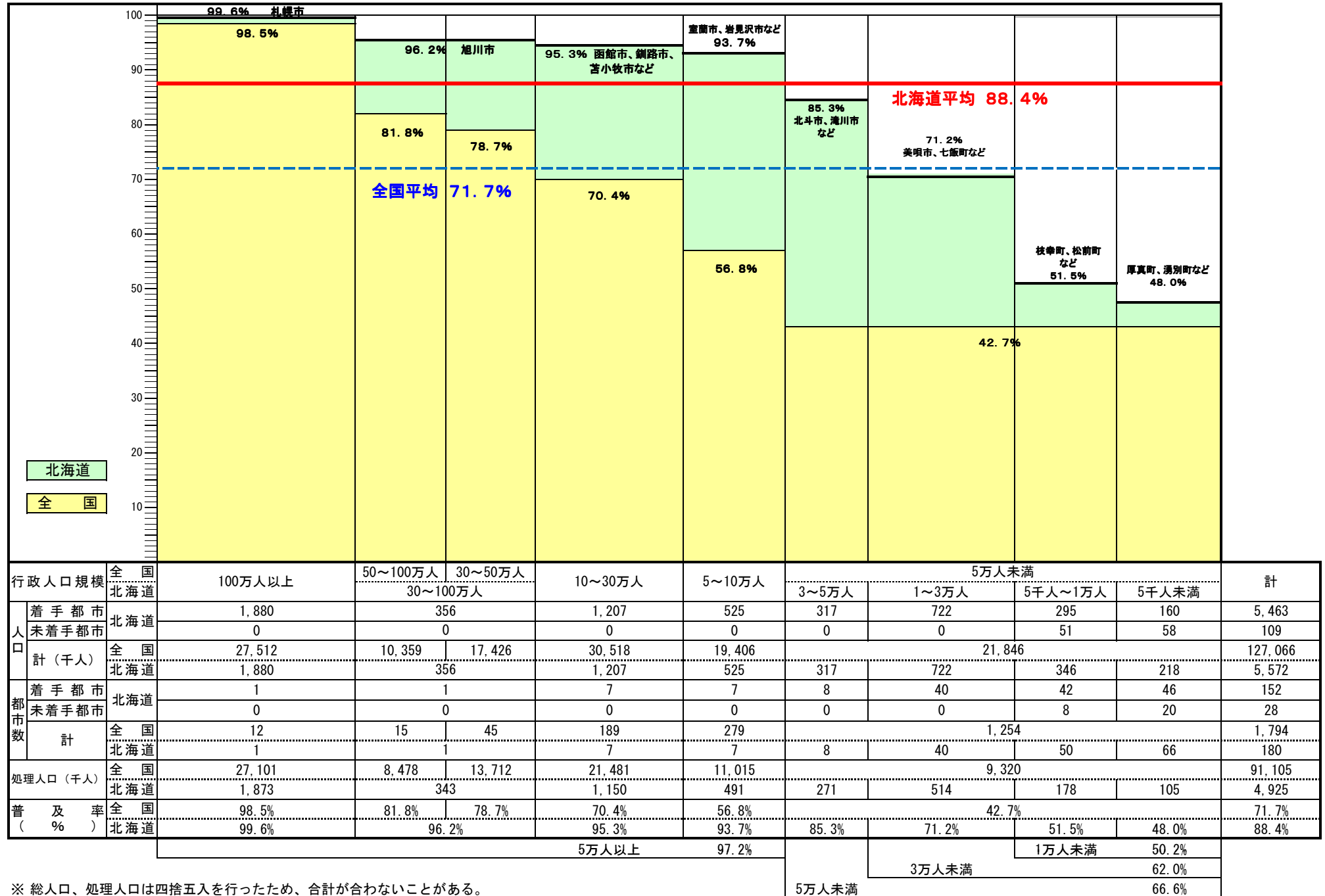
図2 北海道と全国の都市人口規模別下水道処理人口普及状況（平成19年度末）
