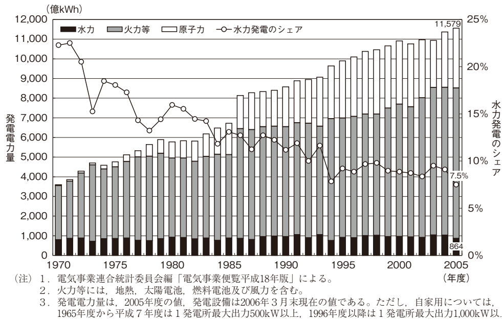
図2-5-1 発電電力量の推移
