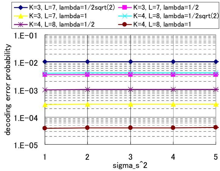
図 6 : カオス信号の分散 \sigma_s^2 に対する誤り率特性
