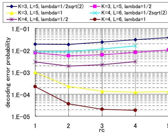
図 7 : カオスシンボル数 r_c に対する誤り率特性
