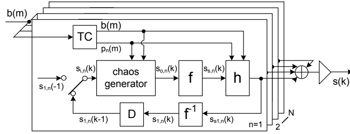
図1：符号化器の構成
