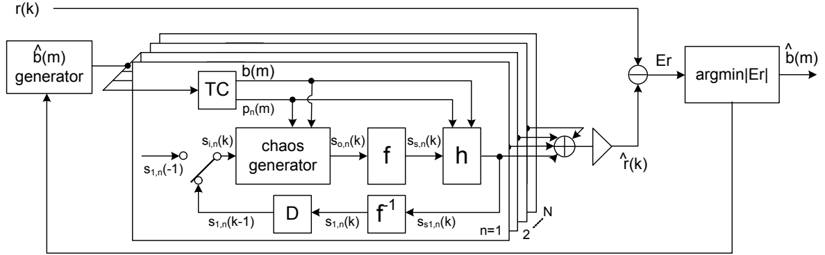
図 3 : 復号器の構成
