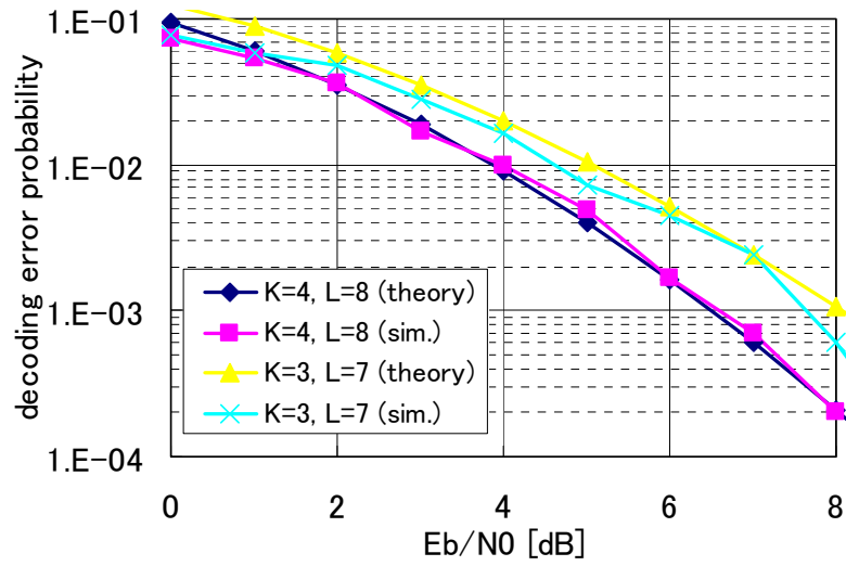
図 5 : 判定誤り率特性
