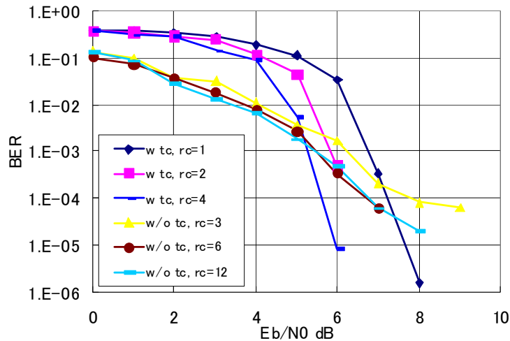
図 10 : 復号誤り率特性
