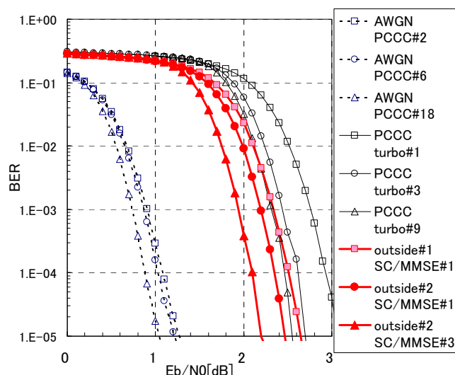
図 1 6 : 提案手法の誤り率特性(位相平均)
