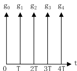
図 1 5 : 静的 5 パス等電力通信路の遅延プロファイル
