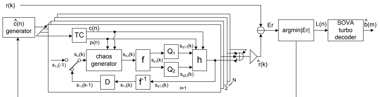
図 9 : ターボ符号接続復号器のブロック図
