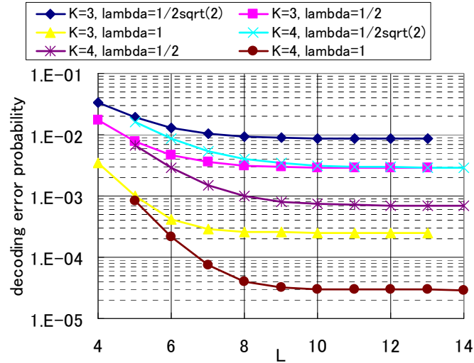
図 8 : 復号拘束長 L に対する誤り率特性
