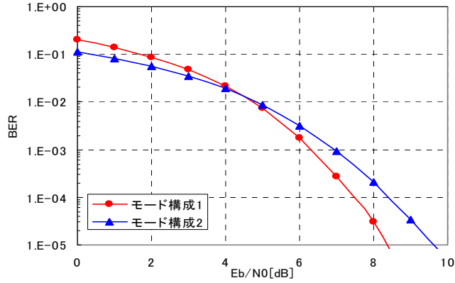
図 1.3 : モード構成の違いによる BER 特性
