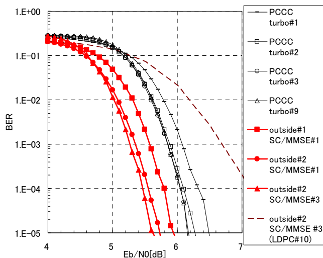
図 1 7 : 提案手法の誤り率特性(位相変化なし)
