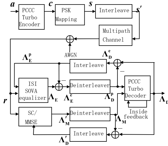
図 1.4 : 提案手法の受信機モデル
