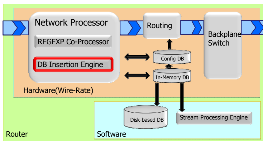
図 1：提案ルータの概要
