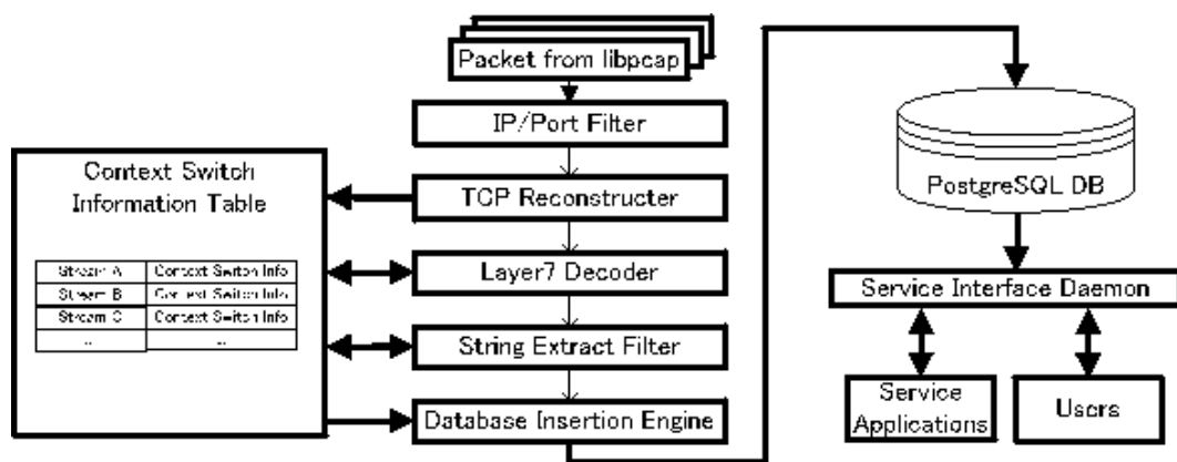
図 2：情報選択，抽出機構
