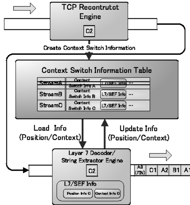
図4：部分 TCP 再構築法
