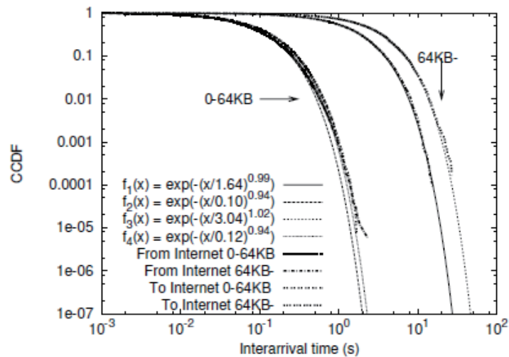
図 6 フロー到着間隔 (測定地点)
