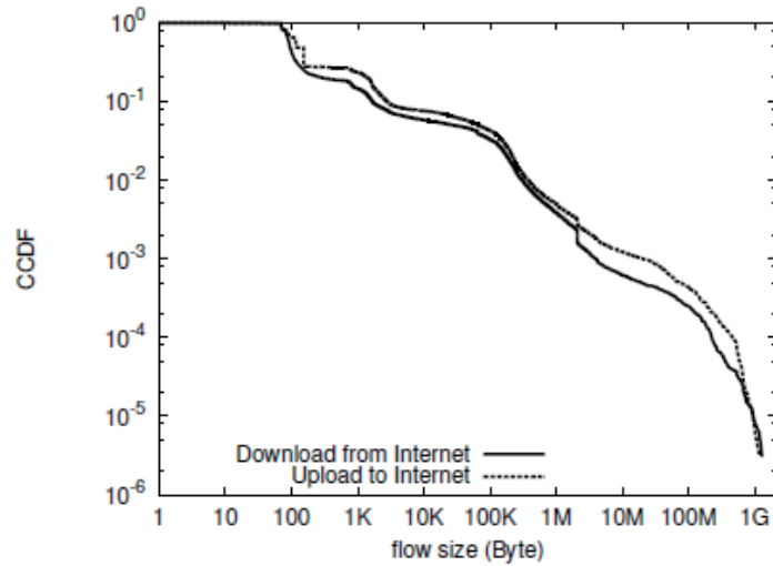
図 5 フローサイズ (インターネットへ, インターネットから)
