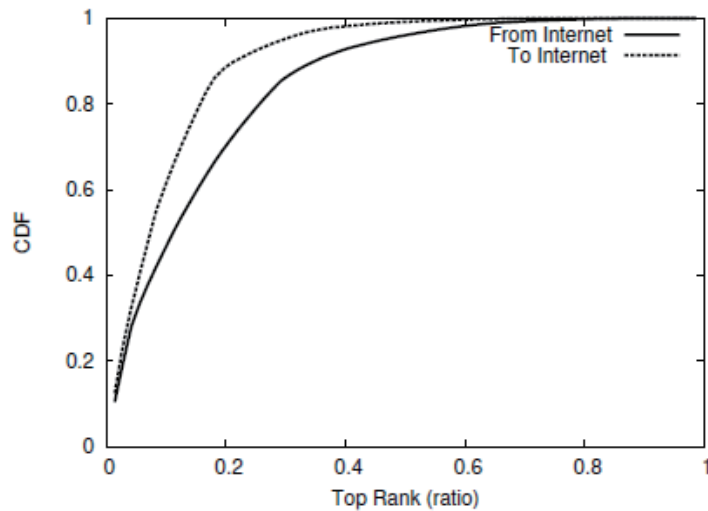
図 7 ピア別の Winny トラフィック量 (72 ホストの上位順, ISP 内)
