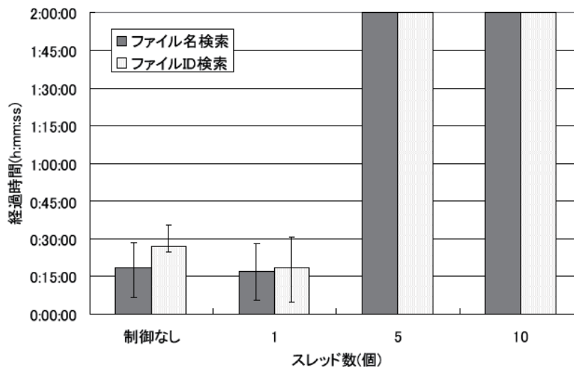
図 13 ファイル ID 検索に対するポイズニングでダウンロードに要した時間
