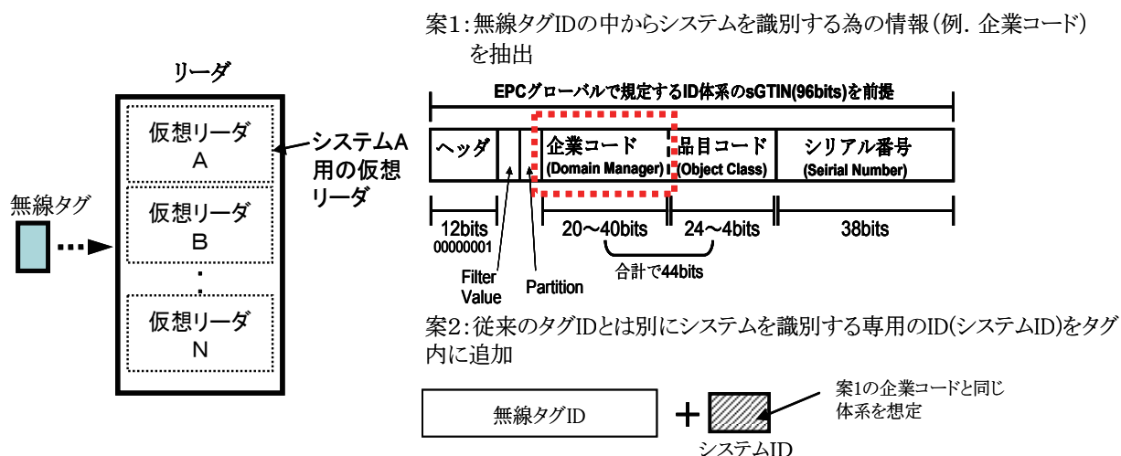
図3. 無線タグと仮想リーダーの連携方式
