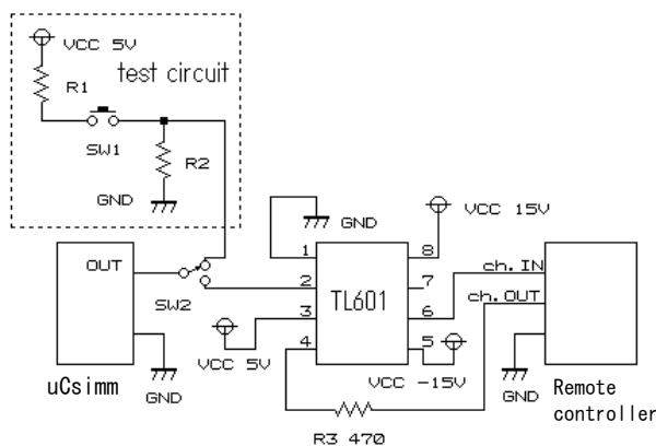
Fig.11 I/O controller.
