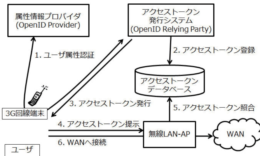
【図 3：公衆無線 LAN サービスシステムの構成図】
