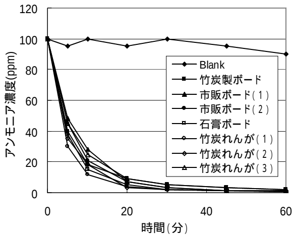
図3 アンモニア吸着性能評価
