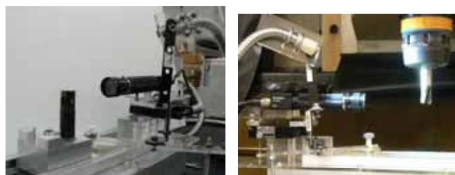
(a) オフライン実験 (b) オンライン実験
