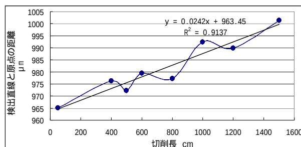
図13 切削長と \rho の関係
