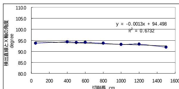
図14 切削長と \theta の関係
