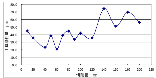
図16 オンラインにおける切削長と工具摩耗量(1)
