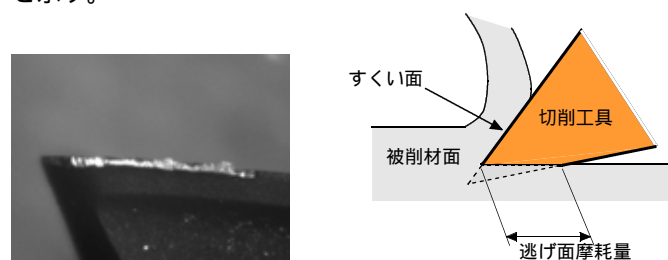
(a) 逃げ面摩耗の写真
