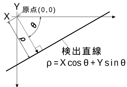
図10 \rho および \theta の定義
