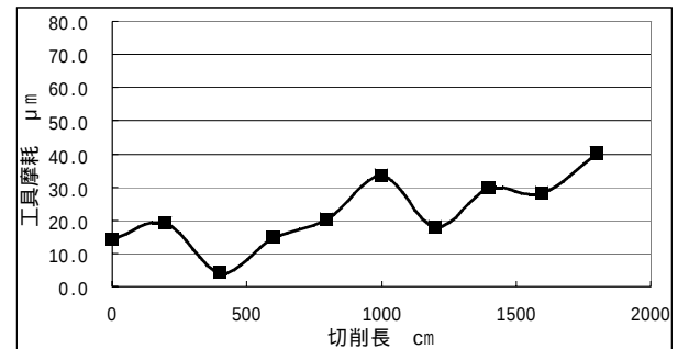
図17 オンラインにおける切削長と工具摩耗量(2)
