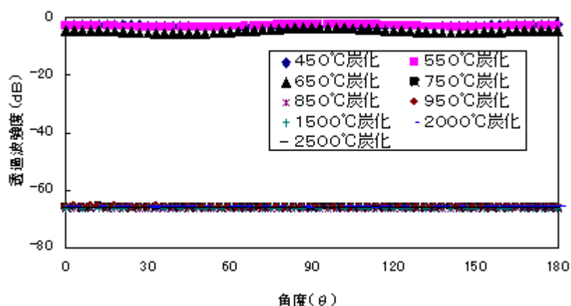
図6 竹炭の35GHzにおける透過波強度の異方性
