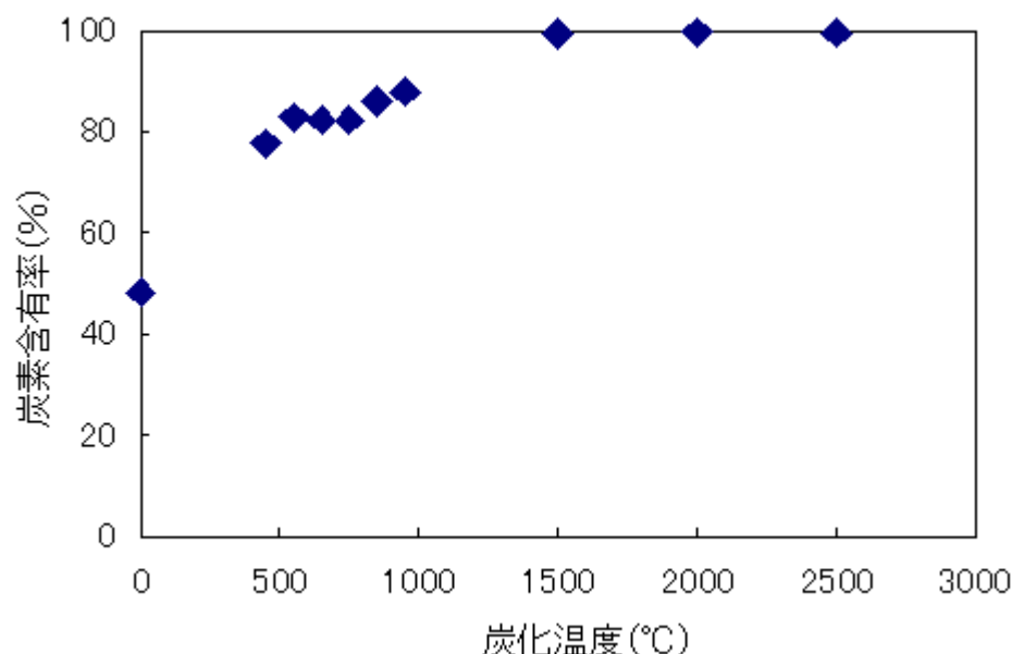
図3 竹炭の炭素含有率に及ぼす炭化温度の影響
