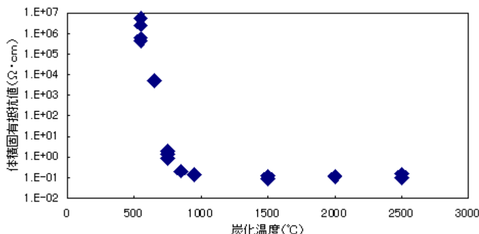
図1 竹炭の体積固有抵抗値と炭化温度の関係
