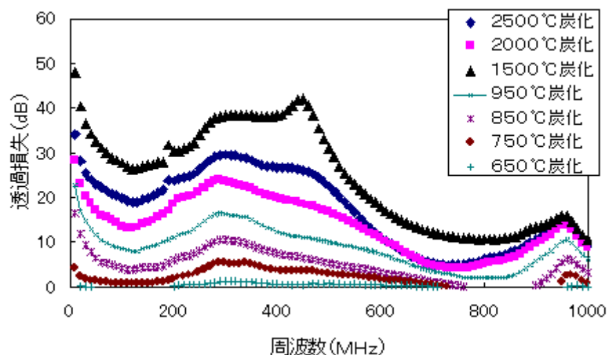
図8 竹炭／エポキシ複合材の透過損失
