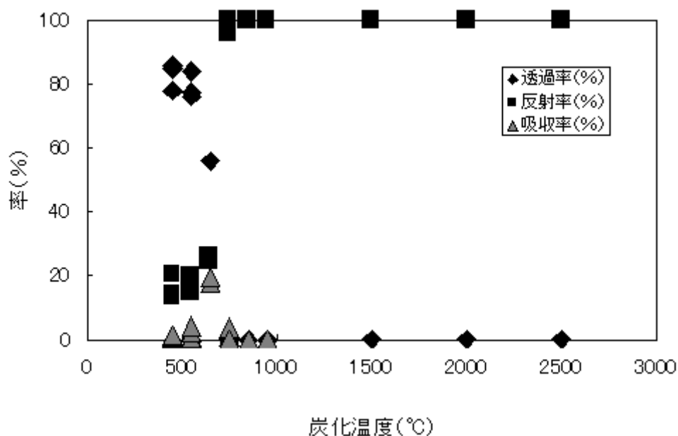
図4 竹炭の導波管内法による測定
