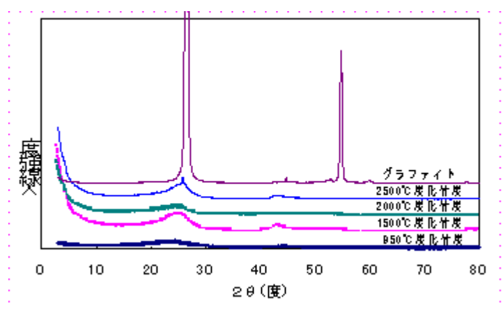
図2 竹炭のX線回折パターン
