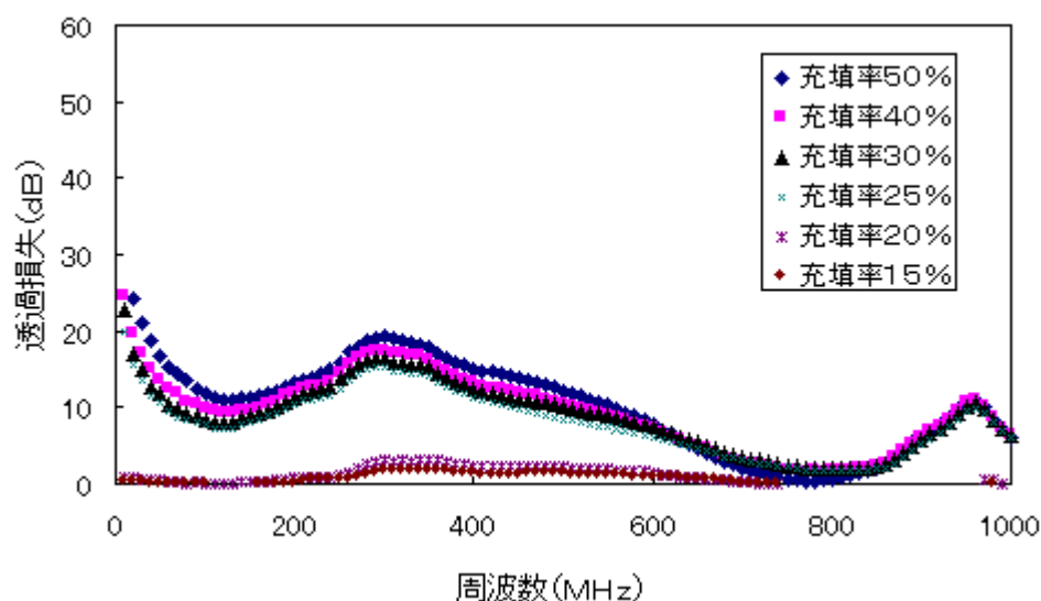
図9 竹炭／エポキシ系樹脂複合体における充填率と透過損失の関係
