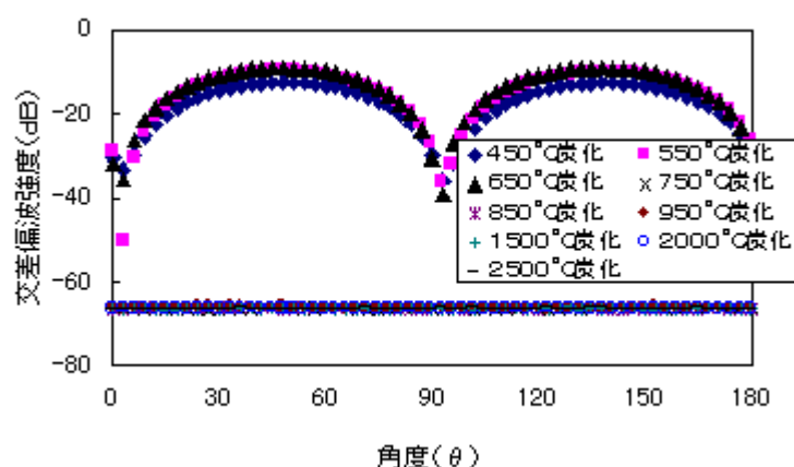
図7 竹炭の35GHzにおける交差偏波強度
