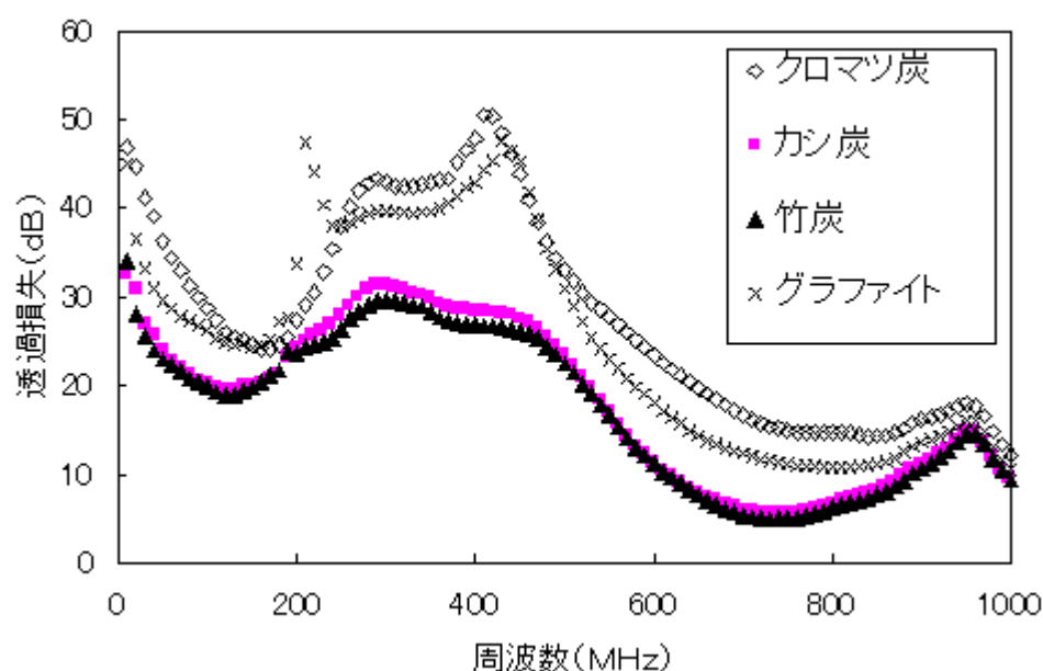
図11 種類の異なる炭化物によるエポキシ系樹脂複合体の透過損失
