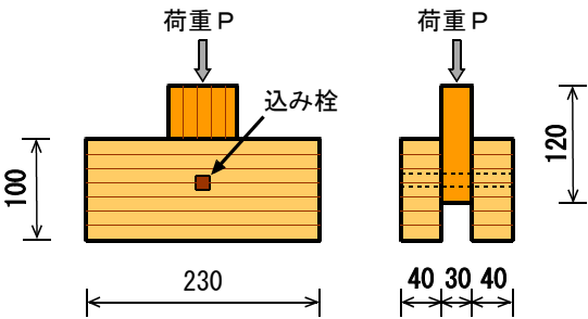
図1 接合部の二面せん断試験方法 (mm)
