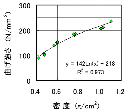
図6 密度と曲げ強さの関係
