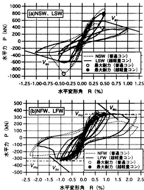
図-3 水平力-水平変形角曲線
