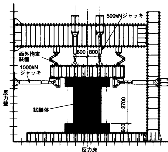
図-2 加力装置 (NFW、LFW)
