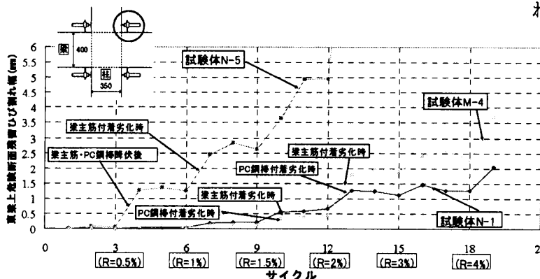
図-9 東梁上危険断面残留ひび割れ幅推移
