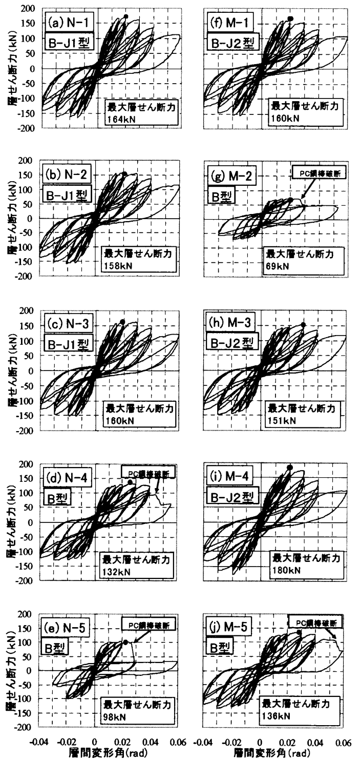
● : 最大層せん断力時 図-5 層せん断力-層間変形角関係
