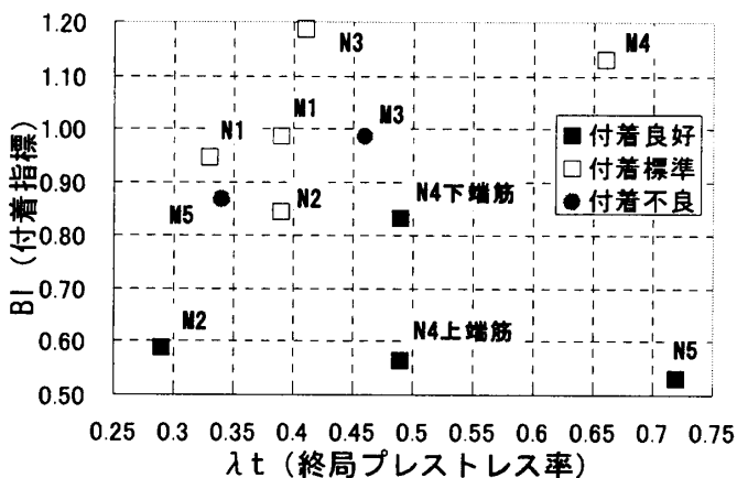
図-2 BI-λt 関係
