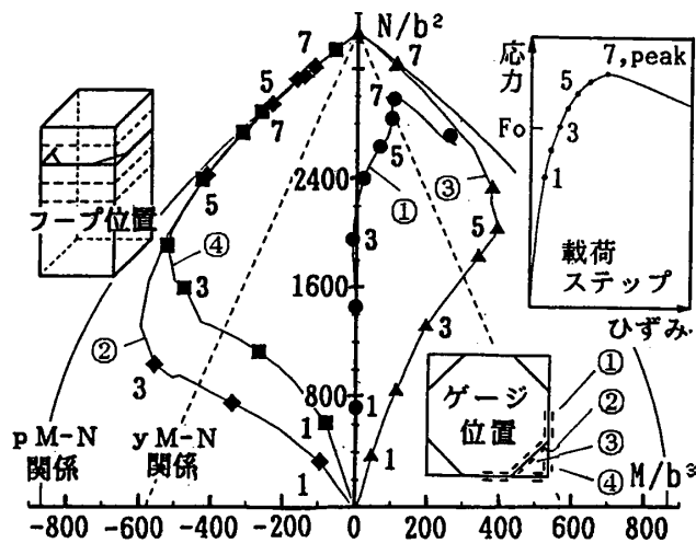
図5 □形横補強筋 M-N相関関係図
