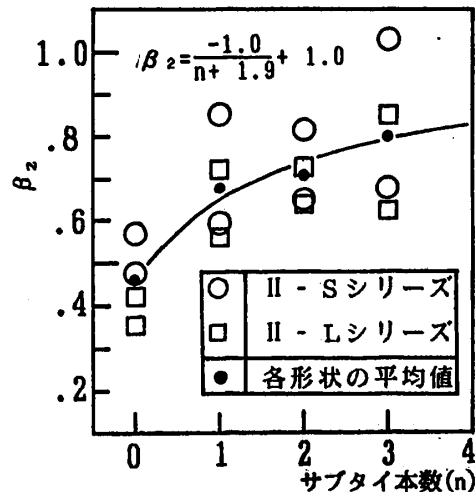
図10 \beta_2 - n 関係
