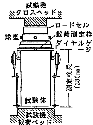
図1 載荷および測定方法
