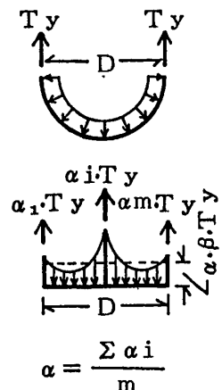
図8 各横補強筋形状での拘束力分布性状
