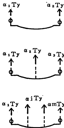
図6 有効軸力係数 \alpha 算定位置
