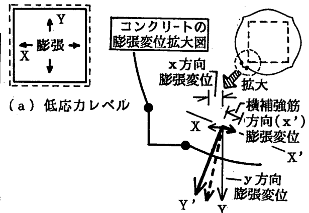
図3 口形横補強筋でのコンクリートの膨張変位
