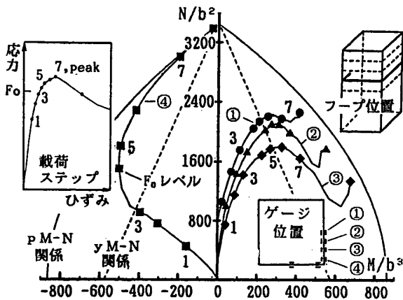
図2 口形横補強筋 M-N 相関関係図
