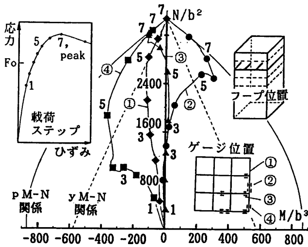
図4 円形横補強筋 M-N相関関係図
