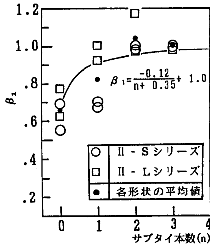
図9 \beta_1 - n 関係
