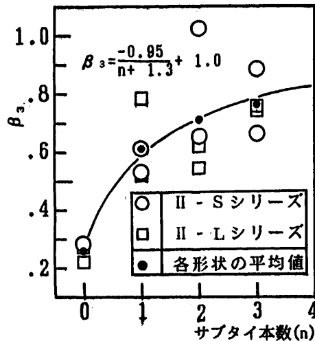
図11 \beta_3 - n 関係
