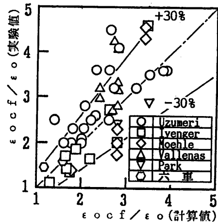
(b) 圧縮強度時ひずみ算定式の検討
