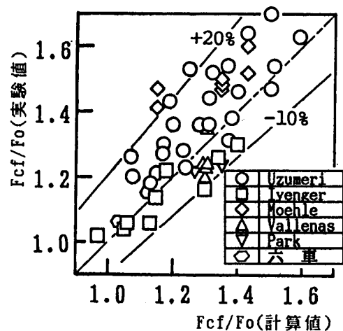
(a) 圧縮強度算定式の検討
