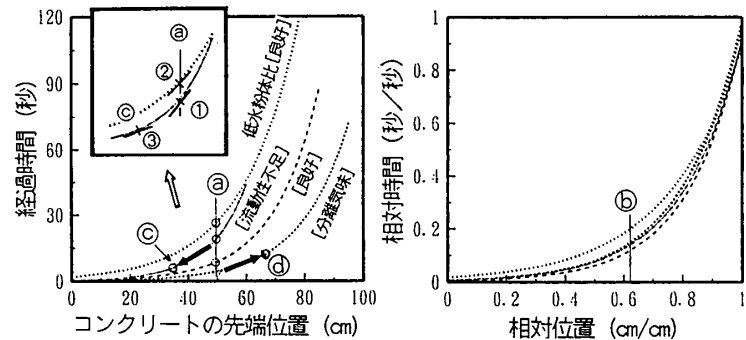
図6 経過曲線上の速度比較
