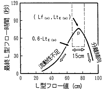
図10 L型フロー試験による管理領域
