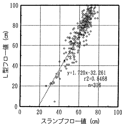
図3 L型フロー値とスランブフロー値の関係
