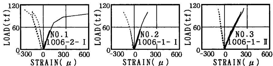
図-17 荷重-コンクリート主ひずみ
