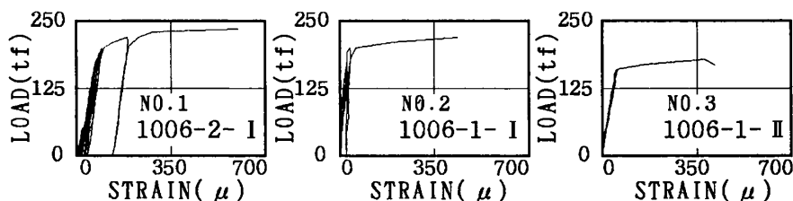
図-18 荷重-円周方向筋ひずみ (外側)
