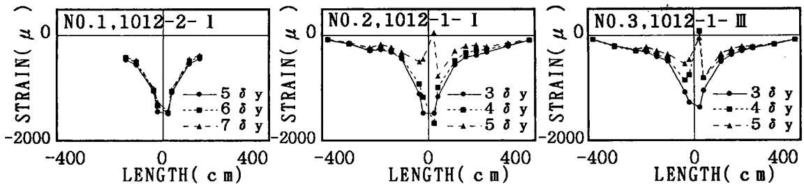
図-9 コンクリート圧縮ひずみ分布
