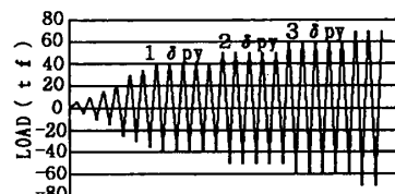
図-3 荷重サイクル
