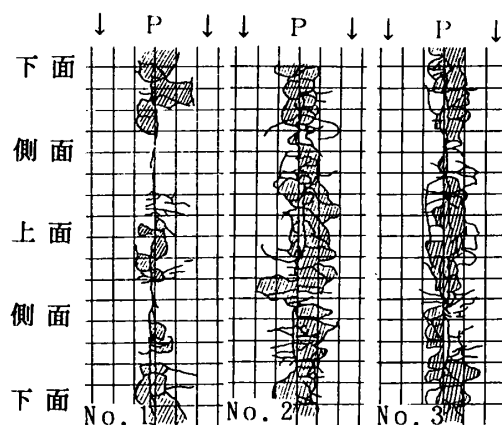
図-6 ひび割れ形状図 (荷重中央部展開図)
