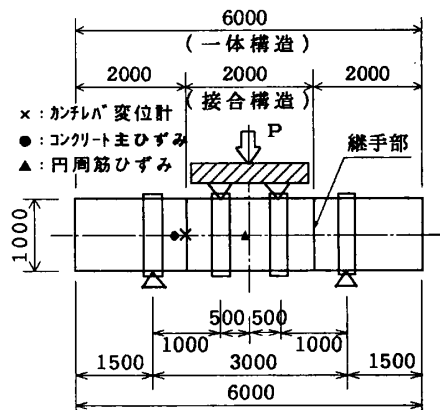
図-4 せん断荷重形式
