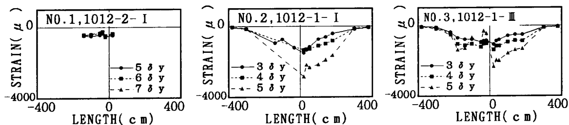
図-8 PC鋼棒圧縮ひずみ分布
