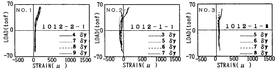
図-11 円周方向筋ひずみ分布 (内側)
