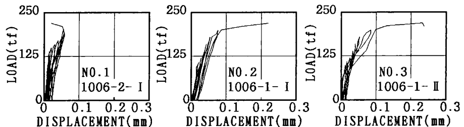
図-16 荷重-カンチレバー変位
