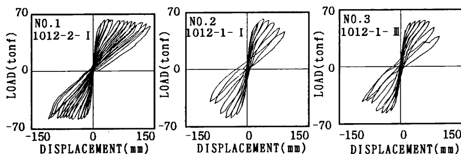
図-7 荷重-変位履歴
