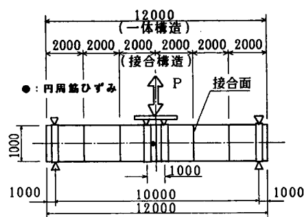
図-2 曲げ荷重形式
