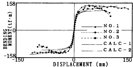
図-15 荷重-変位 (载荷中央点)
