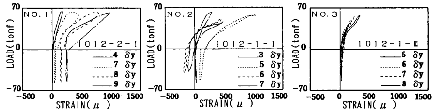
図-10 円周方向筋ひずみ分布 (外側)
