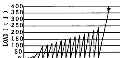
図-4 せん断荷重形式
