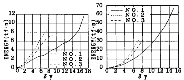
図-12 吸収および累積吸収エネルギー
