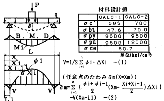
図-13 曲げ変形による変位
