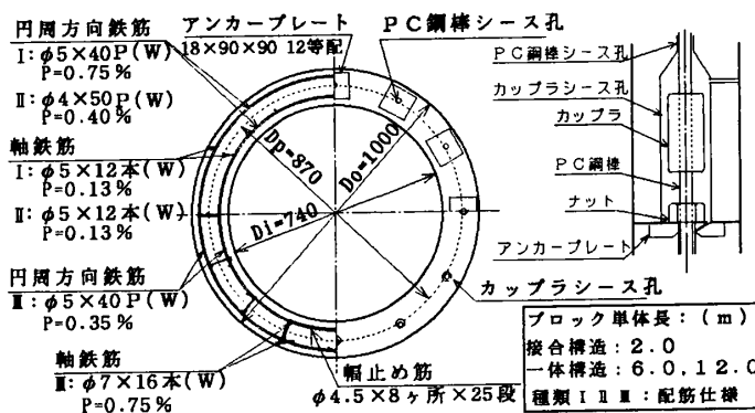
図-1 供試体断面
