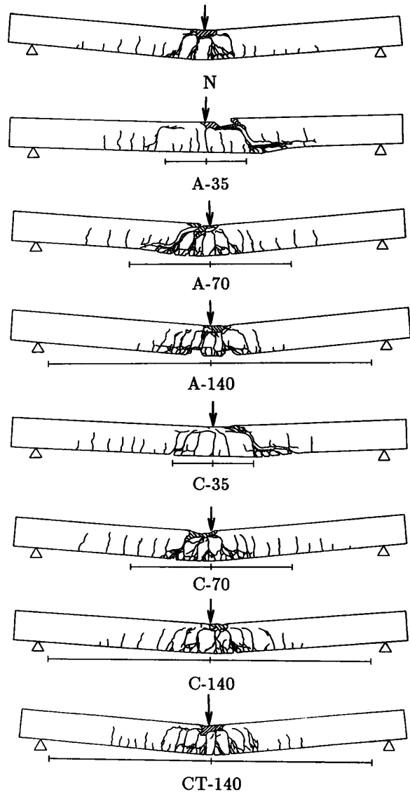
図-6 ひび割れ性状
