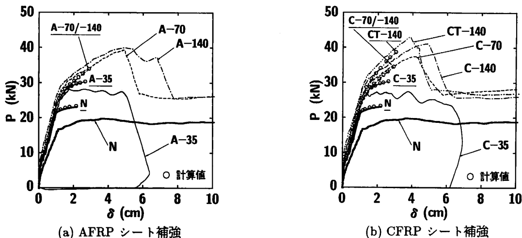
図-2 荷重-変位関係
