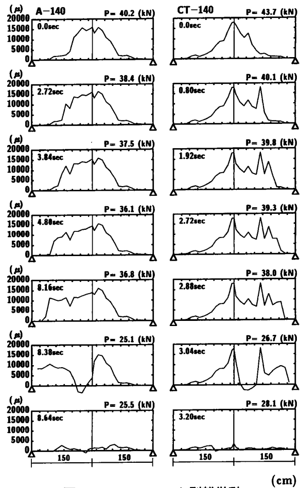
図-5 FRP シート剝離挙動
