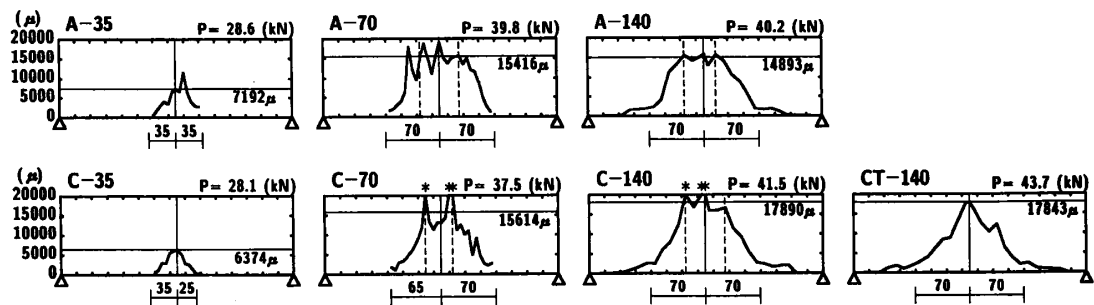
図-4 実測最大荷重時近傍におけるシートの軸歪分布 (cm)
