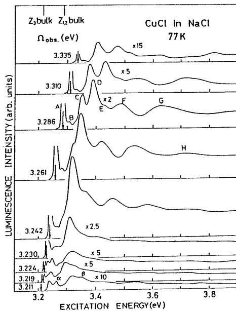
第5図 NaCl中のCuCl微結晶の励起子発光を種々のエネルギー位置で観測した励起スペクトル。矢印で示された \Omega_{obs} は観測エネルギーである。 Z_3, Z_{1,2} \text{ bulk} は、バルク結晶での励起子エネルギー。
