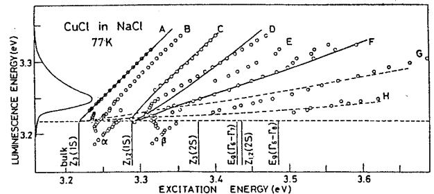
第6図 NaCl中のCuCl微結晶の励起子発光の励起スペクトルに現れたA~Hのピークエネルギーと観測している発光エネルギーとの関係。○印は実験点で、曲線は \langle 111 \rangle 方向の量子サイズ効果を受けた励起子状態に基づく計算値である。下欄の縦棒はバルク結晶における種々の励起子状態のエネルギー位置を示す。
