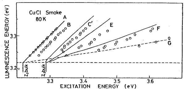
第7図 \rightarrow ガス中蒸発法によるCuCl微結晶の励起子発光の励起スペクトルのピークエネルギーと観測している発光エネルギーとの関係。○印は実験点で、曲線は第6図と同じ。
