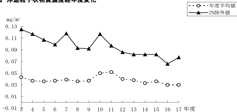
第Ⅲ-10図 浮遊粒子状物質濃度経年度変化
