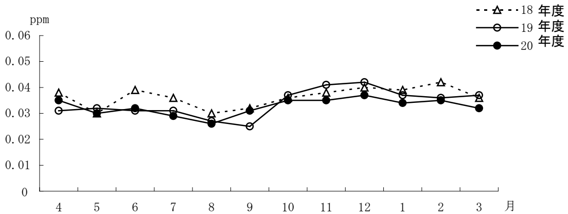
第Ⅲ-12表 二酸化窒素濃度月平均値(自動車排出ガス測定局)
